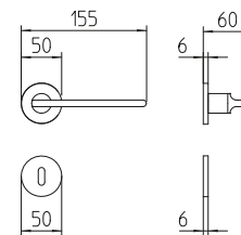
1751 maniglia per porta con rosetta door handle on rose
