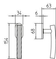
1732/DK martellina dk drehkipp system
