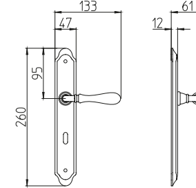
1420 con piastra door handle on backplate
