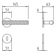
1731 maniglia per porta con rosetta door handle on rose
