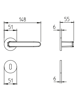
1871 maniglia per porta con rosetta door handle on rose
