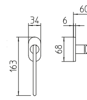
1752/DK martellina dk drehkipp system
